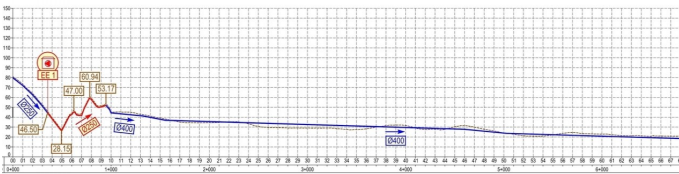
ESQUEMA HIDRÁULICO - SOLUÇÃO A Esc.: H=1:20 000; V=1:10 000
